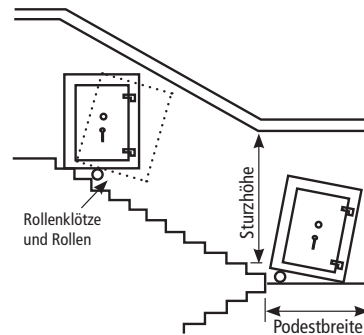
6. Treppe 180° abgewinkelt mit Podest
