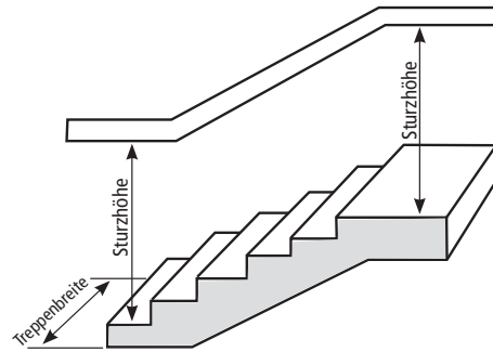
2. gerade Treppe mit Unterzug
